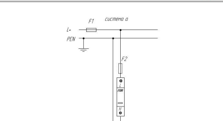
Схема подключения ГСВ1 (C) для сети постоянного тока типа TN-C
