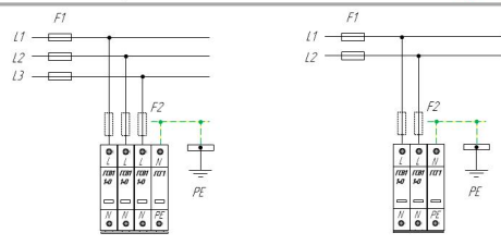
Схема подключения ГСВ1 1-0 (C) ГСГ1 для сети с системой заземления типа IT
