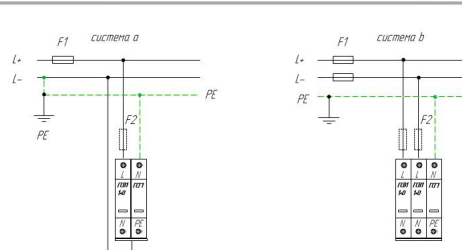
Схема подключения ГСВ1 1-0 (C) ГСГ1 для сети постоянного тока типа TN-S
