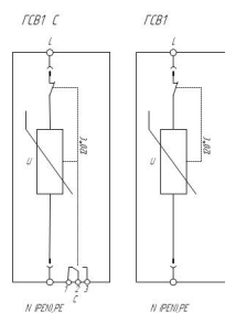
Схемы электрические принципиальные УЗМП серии ГРОЗДОСТОН® ГСВ1 (C)
