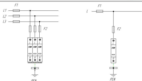
Схема подключения ГСВ1 (C) для сети с системой заземления типа TN-C
