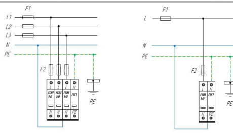
Схема подключения ГСВ1 1-0 (C) ГСГ1 для сети с системой заземления типа TN-S
