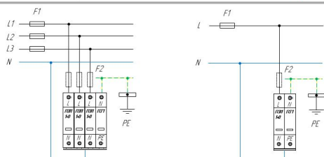
Схема подключения ГСВ1 1-0 (C) ГСГ1 для сети с системой заземления типа TT
