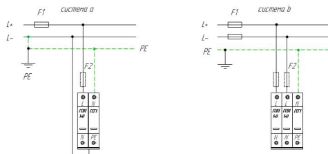
Схема подключения ГСВ1 1+0 (C) ГСГ1 для сети постоянного тока типа TN-S
