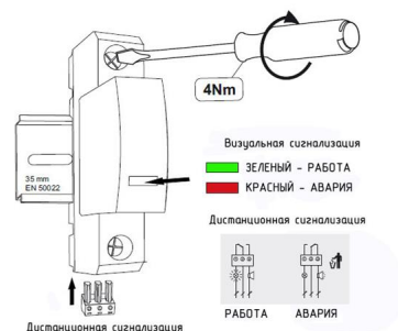
Визуальная и дистанционная сигнализация УЗИП серии ГСВ1 (C)
