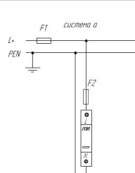
Схема подключения ГСВ1 (L) для сети постоянного тока типа TN-C
