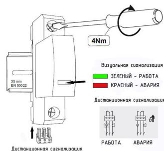
Визуальная и дистанционная сигнализация УЗИП серии ГСВ1 (L)
