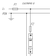
Схема подключения ГСВ1 (С) для сети постоянного тока типа TN-C
