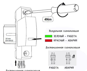
Визуальная и дистанционная сигнализация УЗИП серии ГСВ1 (С)
