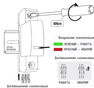
Визуальная и дистанционная сигнализация УЗИП серии ГСВ1 (L)
