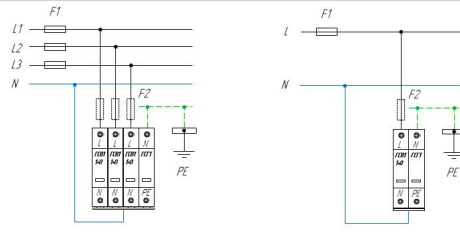
Схема подключения ГСВ1 1-0 (L) ГСГ1 для сети с системой заземления типа TT
